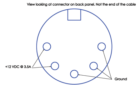
5 pin DIN 12 V Transport Supply
